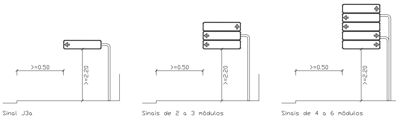
Figura 3.5 - Colocação vertical dos sinais de direcção J3 - indicação de âmbito urbano
