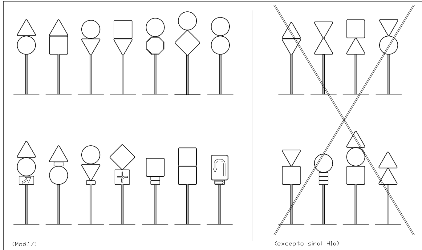
Figura 3.8 – Exemplos de conjugação de “sinais de código” num mesmo suporte
