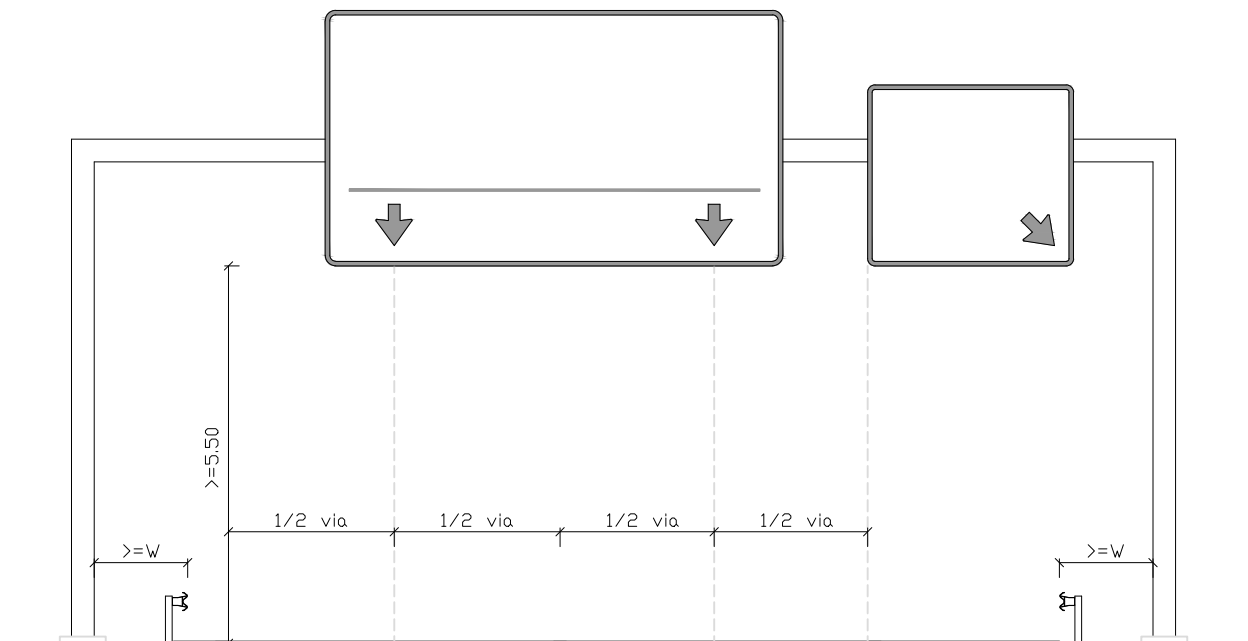
Figura 3.3 - Colocação vertical de sinais colocados por cima da via - exemplo para E1 + E2
