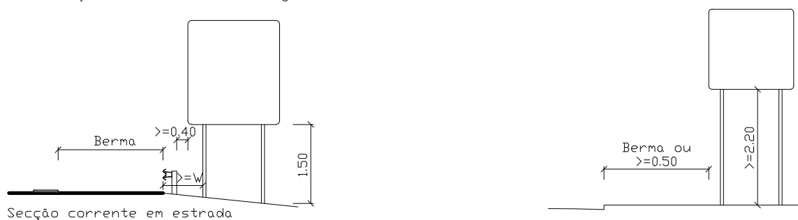
Figura 3.2 - Colocação vertical de sinais de grandes dimensões
