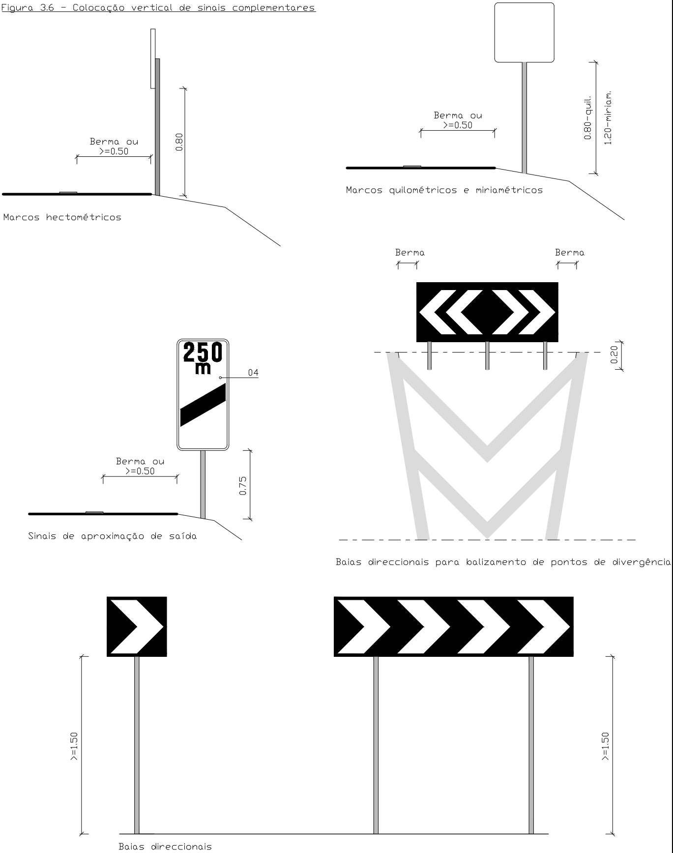
Figura 3.6 - Colocação vertical de sinais complementares
